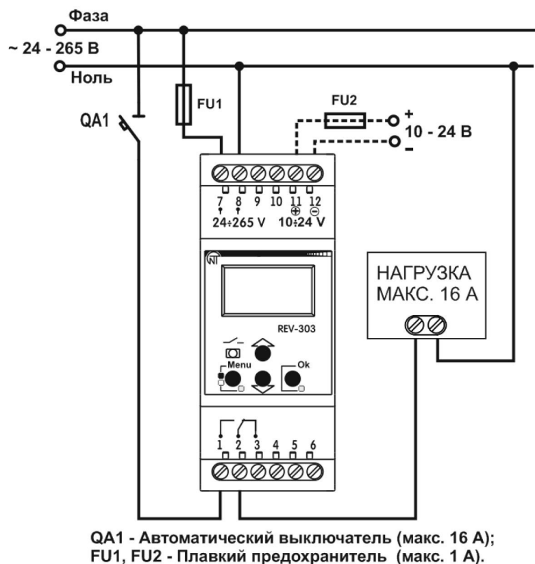
Рисунок 5.1 – Схема подключения REV-303
